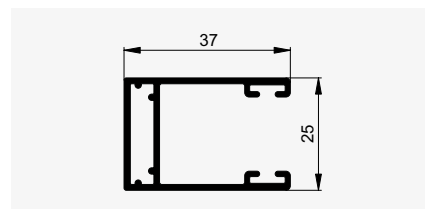
Für Stab DP 54
